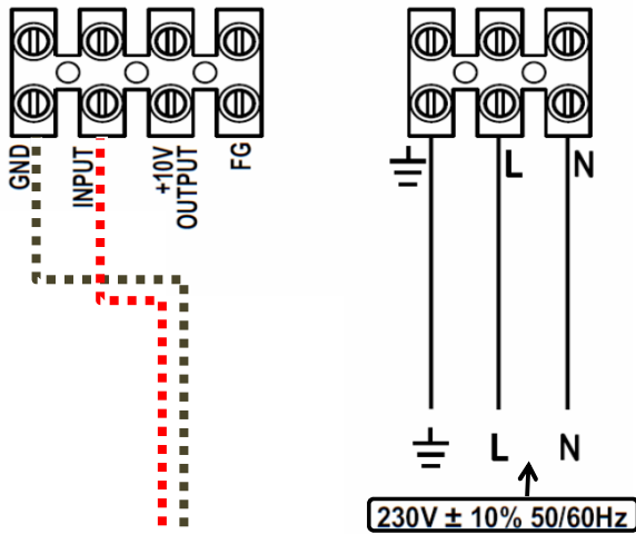
Aansluitschema buisventilator :
