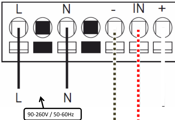
Aansluitschema buisventilator :
