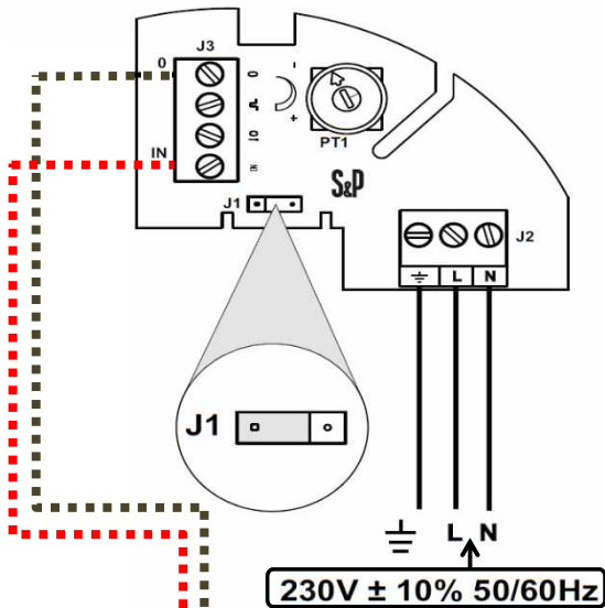
Aansluitschema buisventilator :
