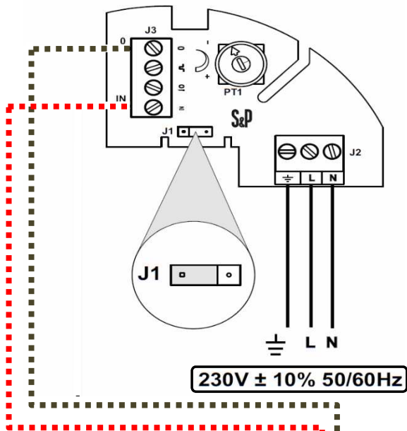
Aansluitschema buisventilator :
