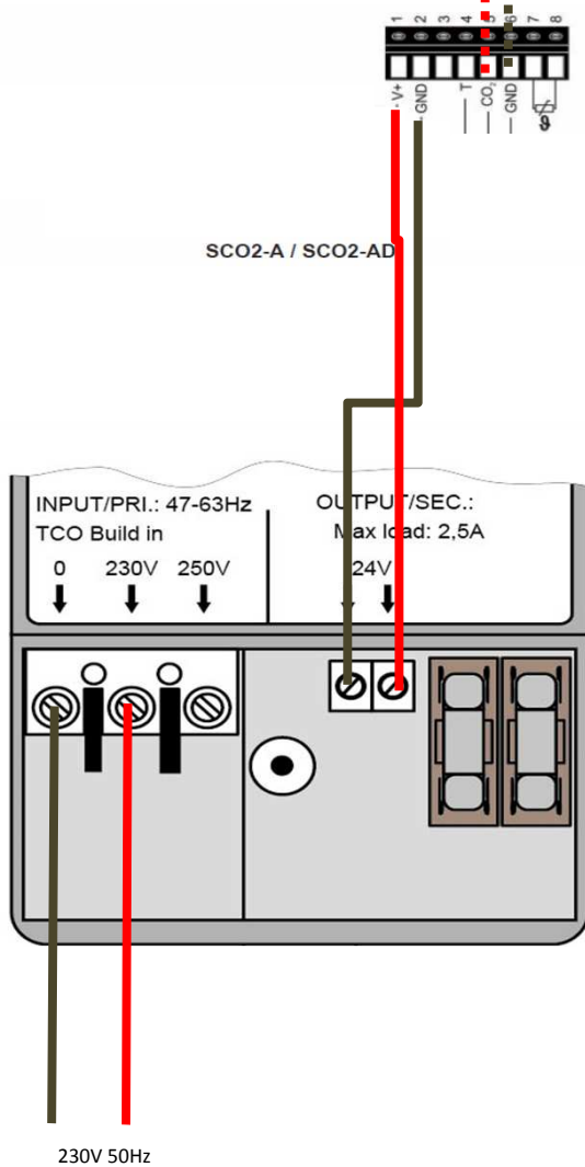
Aansluitschema TRAF060 :
