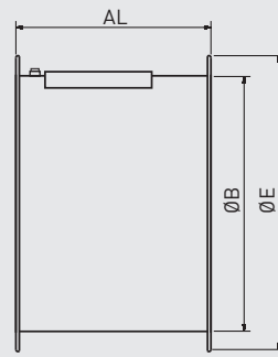
Lange behuizing (LP) TGT 400 tot 800
