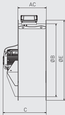
Korte behuizing (C en CK) - tot IEC 200 Alleen met aansluitdoos (CK) - vanaf IEC 225
