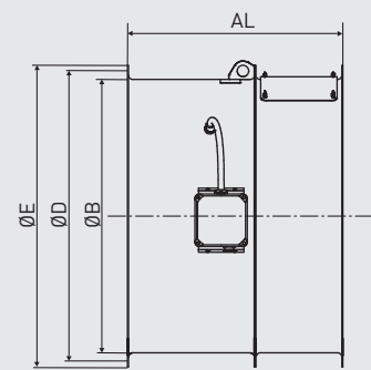
Lange behuizing (LPK) TGT 900 tot 1250
