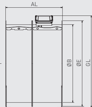
Lange behuizing (LP, LK en LPK) - tot IEC 200 Alleen met aansluitdoos (LK en LPK) - vanaf IEC 225
