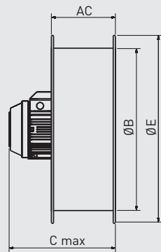
Korte behuizing (C) TGT 400 tot 1250
