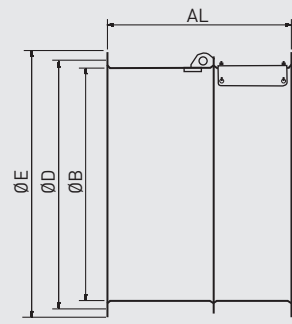
Lange behuizing (LP) TGT 900 tot 1250
