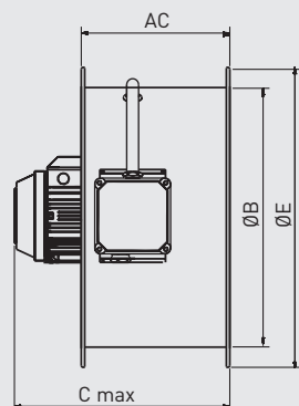
Korte behuizing (CK) TGT 400 tot 1250
