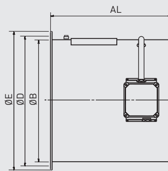
Lange behuizing (LK en LPK) TGT 400 tot 800
