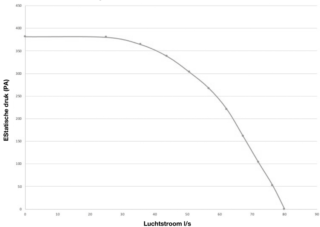
energisava 260 Statische druk- luchtstroom
